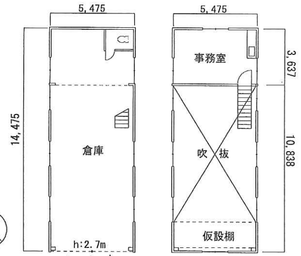
2階平面図
