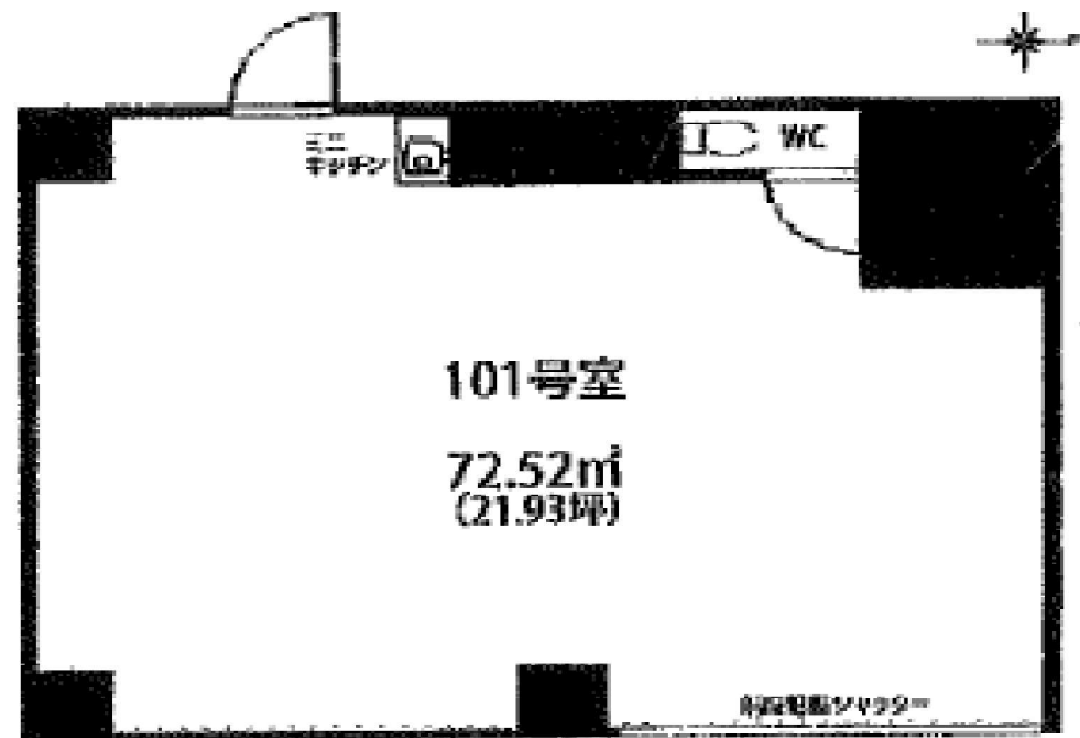
1階平面図 公道8.0m
