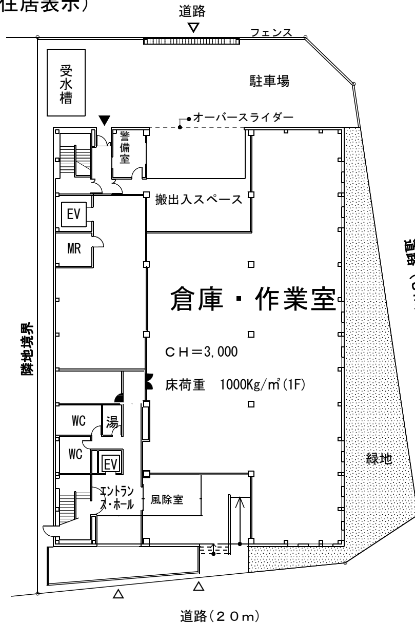
1階平面図
