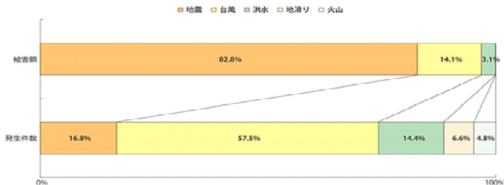
第2-4-3図 日本における自然災害被害額の災害別割合
